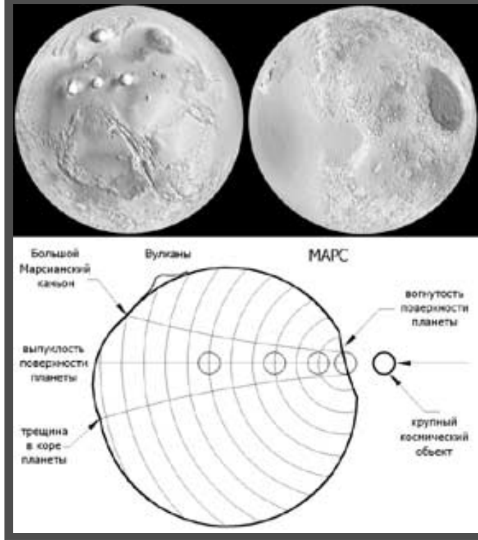
Кратеры, долины Маринер и впадина на противоположной стороне Марса. Картина высот.
