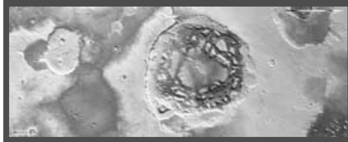
Кратеры, долины Маринер и впадина на противоположной стороне Марса. Картина высот.
