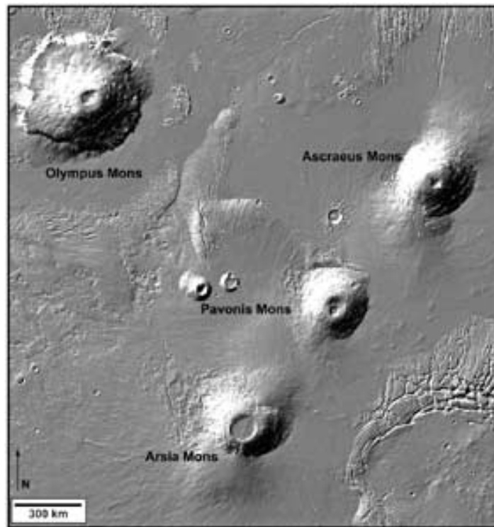
Фото: Интересная геометрия расположения вулканов на Марсе
