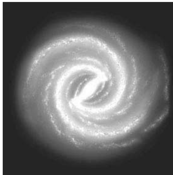
Рис 1а. Художественная интерпретация Млечного Пути, наблюдаемого сверху точки северного полюса. Фото и интерпретация из статьи «Млечный путь» ( https://v-kosmose.com/galaktiki-vselennoi/mlechniy-put/ )
